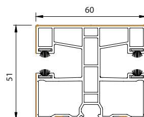
prowadnica podzielowa
