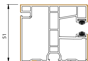
prowadnica jednostronna
