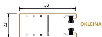
prowadnica jednostronna
