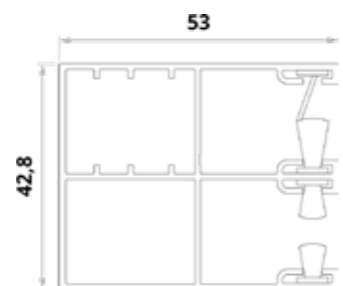
Prowadnica jednostronna z moskitierą (dla lameli H37 i H42).
