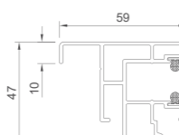
Prowadnica (ALU) jednostronna - RSW A927
