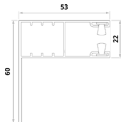
Prowadnica kąтова (dla lameli H37 i H42).
