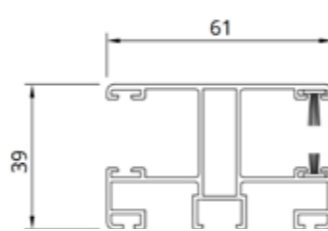
Prowadnica (ALU) jednostronna / dwustronna 01130903BL
