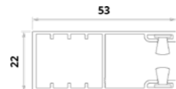
Prowadnica jednostronna (dla lameli H37 i H42).
