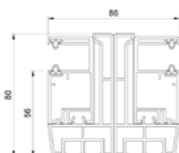
Prowadnica (PVC) podziałowa - RS rewizja od wewnątrz. MK933 + MK9730
