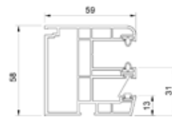
Prowadnica (PVC) jednostronna + MKT* - RS rewizja od wewnątrz. MK8110
