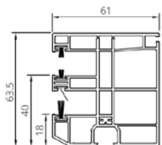
Prowadnica (PVC) jednostronna + MKT*. R0003
