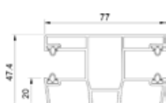
Prowadnica (PVC) podziałowa - RS rewizja od wewnątrz. MK939
