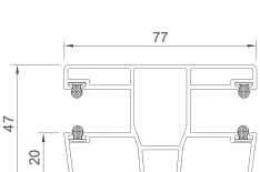
Prowadnica (ALU) dwustronna - RSW A939
