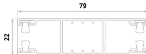
Prowadnica dwustronna (dla lameli H37 i H42).
