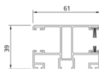
Prowadnica (ALU) jednostronna / dwustronna 01130903BL
