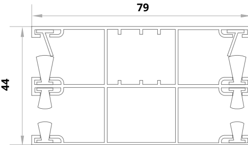
Prowadnica (ALU) dwustronna + MKT
