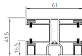
Prowadnica (PVC) dwustronna MAXI. 011309029
