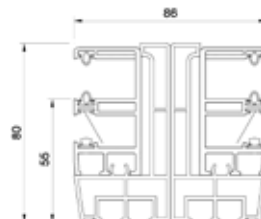
Prowadnica (PVC) podziałowa + MKT* - RS rewizja od zewnątrz. MK8120 + MK9730
