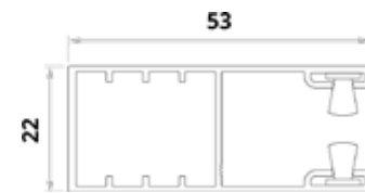
Prowadnica jednostronna (dla lameli H37 i H42).
