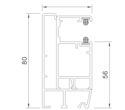
Prowadnica (ALU) jednostronna - RSZ A973+A933
