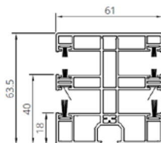
Prowadnica (PVC) dwustronna + MKT*. R0004
