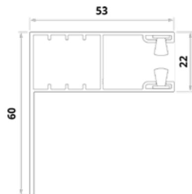
Prowadnica kątowna (dla lameli H37 i H42).
