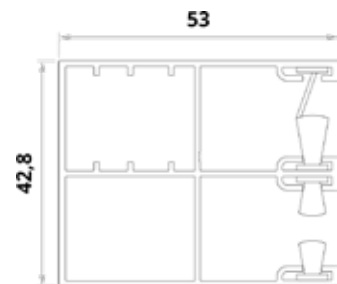
Prowadnica jednostronna z moskitierą (dla lameli H37 i H42).
