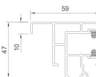
Prowadnica (ALU) jednostronna - RSW A927
