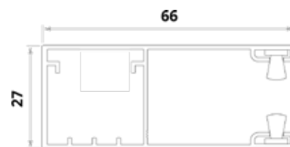
Prowadnica jednostronna (dla lameli H55).
