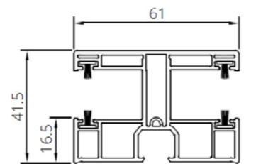
Doppel Führungsschiene (PVC) MAXI. 011309029
