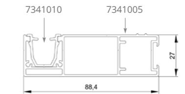
Standardmäßig eiseitige Führungsschienen zum ZF-A.
