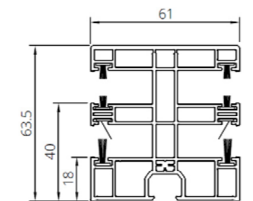
Doppel Führungsschiene (PVC) + INS*. R0004
