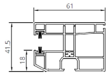
Einseitige Führungsschiene (PVC) MINI. R0001
