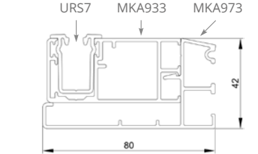
Standardmäßig eiseitige Führungsschienen zum ZF-S.
