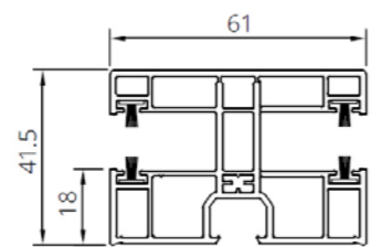
Doppel Führungsschiene (PVC) MINI. R0002
