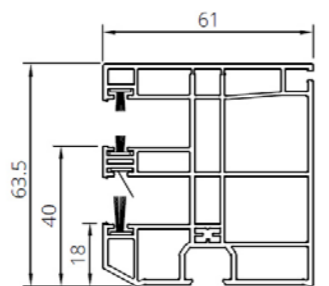
Einseitige Führungsschiene (PVC) + INS*. R0003
